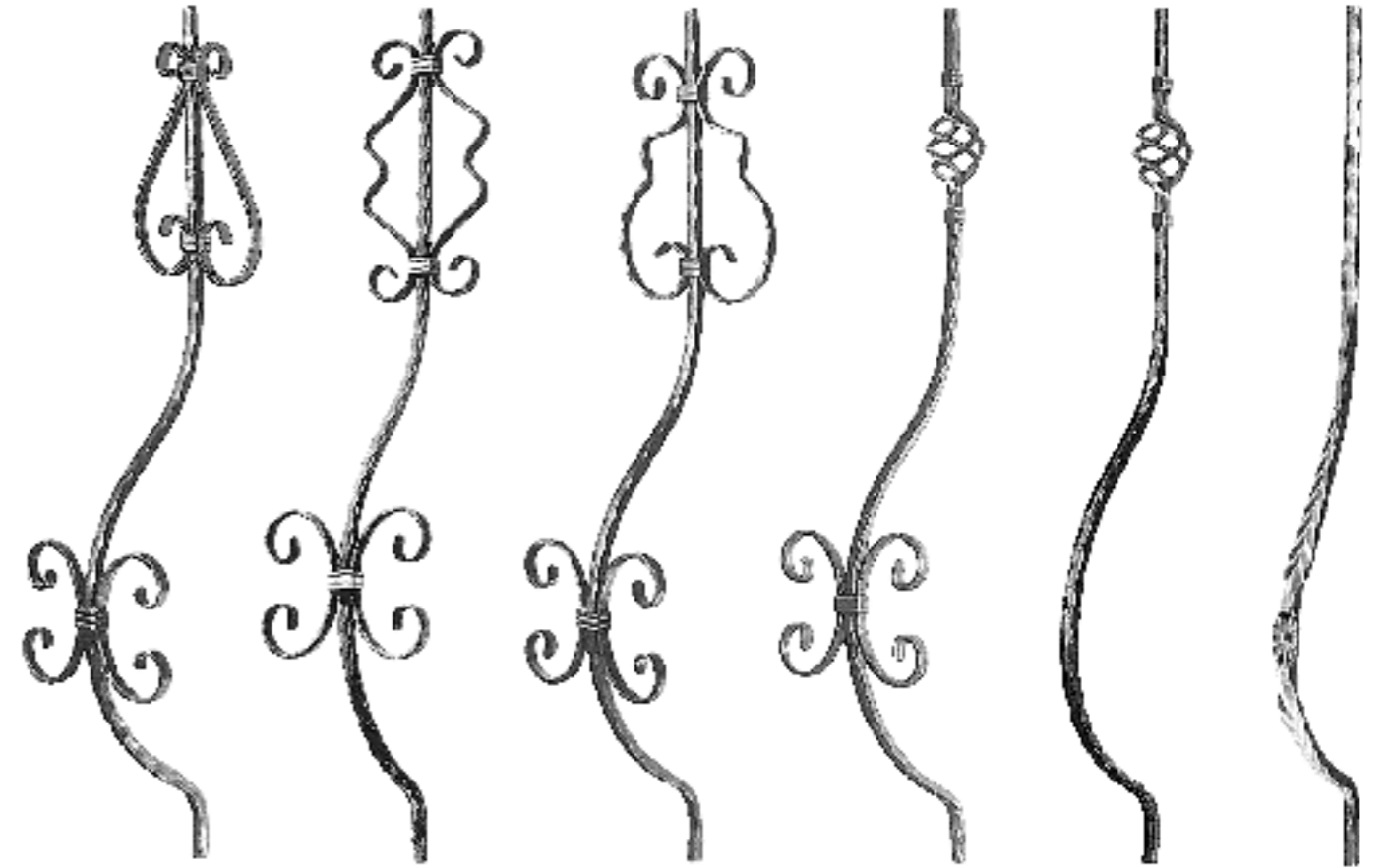
C-730 18x58,5x14 1,84kg. C-749 16x58,5x14 1,89kg. C-750 19x58,5x14 1,92kg. C-752 16x54x14 1,48kg. C-753 5,5x12,5x14 1,11kg. C-755 3x80x15 1,00kg.
