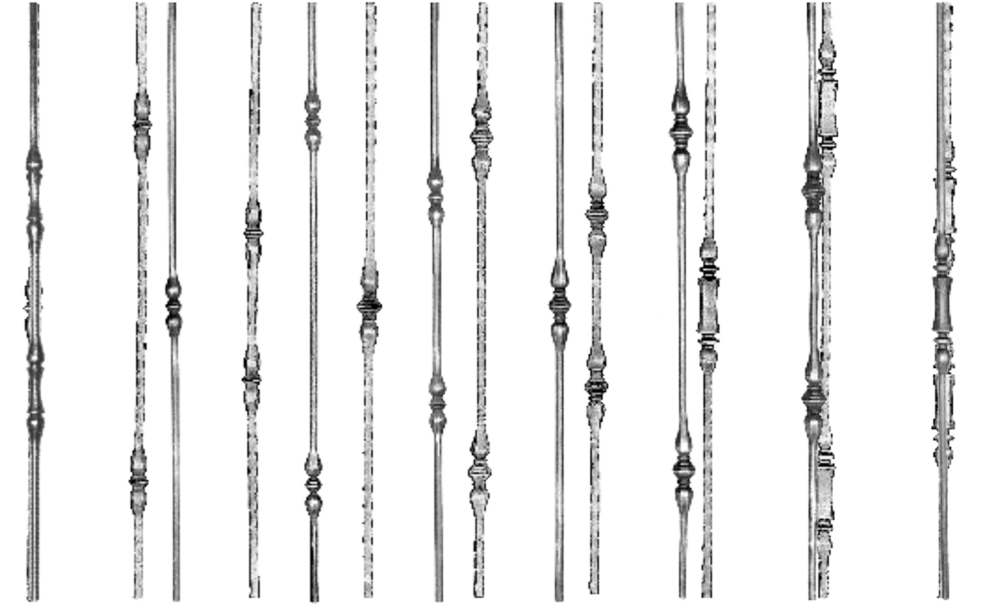
SD-107 2,5x40 1,00kg. SD-307 2,5x50 1,27kg. SD-108 2,5x50 1,27kg. SD-208 2,5x34 1,27kg. SD-208 2,6x57 1,02kg. SD-109 3x12 1,14kg. SD-308 2,6x34 1,02kg. SD-209 3x58 1,44kg. SD-110 3x13 0,94kg. SD-309 3x40 1,44kg. SD-210 3x58 1,17kg. SD-111 3,5x20 1,33kg. SD-311 3,5x65 1,17kg. SD-211 3,5x65 1,17kg. SD-311 3,5x9x20 1,80kg. SD-311 3,5x9x20 1,80kg.
