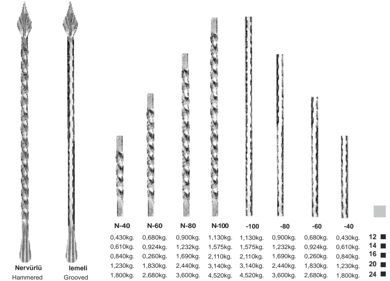
K-100-3 1,29kg. K-100-2 1,21kg. K-100-1 1,17kg. K-80-3 1,08kg. K-80-2 0,99kg. K-80-1 0,95kg. K-60-2 0,79kg. K-60-1 0,70kg. K-40-1-O 0,50kg. K-40-1-Ç 0,50kg.
