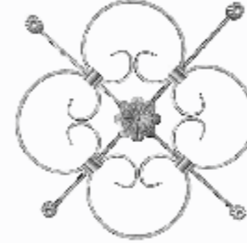
P-132 29,5x29,5 1,38 kg 6x12
