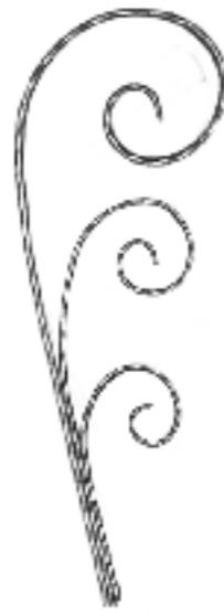
P-312 15x42 0,71kg. 12x6
