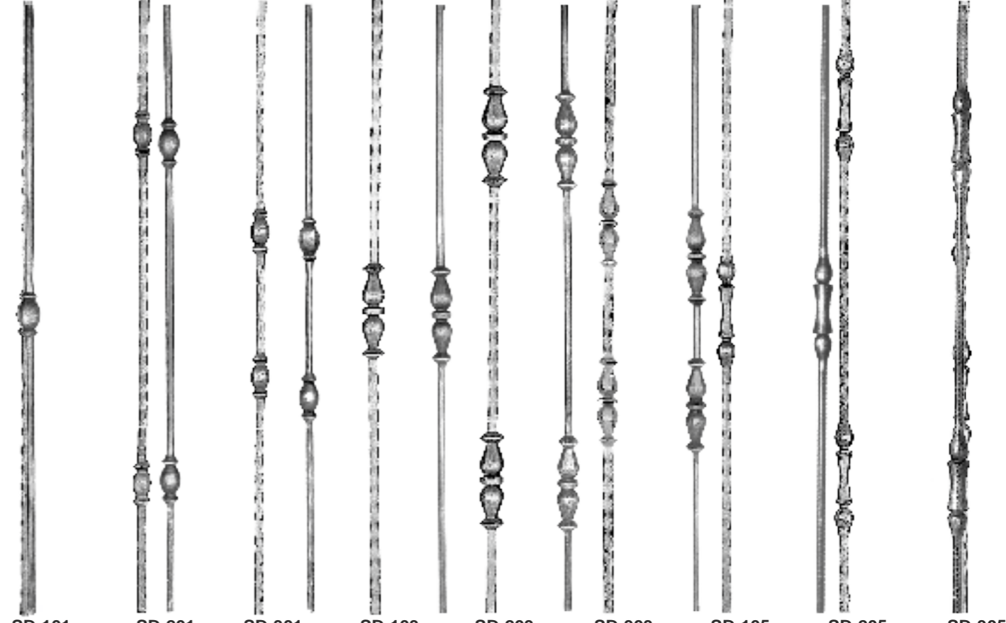
SD-102 3x6,5 0,86kg. SD-202 3x5,5 1,28kg. SD-304 3x30 1,28kg. SD-302 3x30 1,07kg. SD-103 3x13 1,24kg. SD-104 3x13 1,12kg. SD-203 3x58 1,65kg. SD-204 3x58 1,54kg. SD-303 3x40 1,65kg. SD-305 3x40 1,54kg. SD-105 2,5x13,5 1,03kg. SD-205 2,6x13,5 0,84kg. SD-305 2,5x40 1,00kg.
